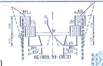
[工程圖]
